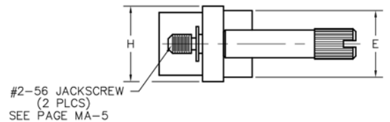
RECEPTACLE
