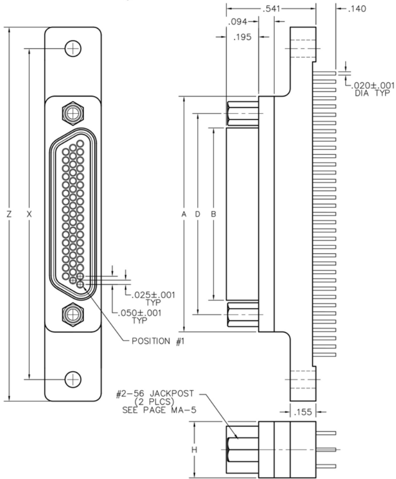
RECEPTACLE
